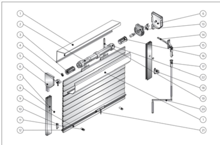
Рисунок 1.6 Роллета с редукторным (воротковым) приводом и съёмным воротком. Масса полотна до 35 кг.
